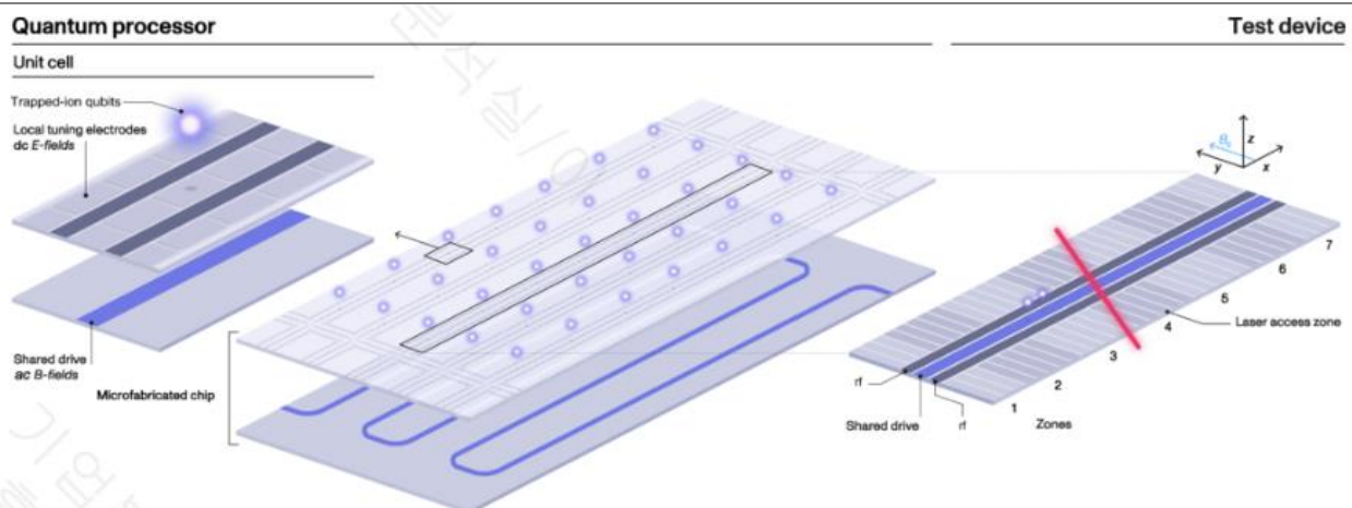
도표 2. 전자/전류 방식 이온트랩 양자컴퓨터 예시 도식도
